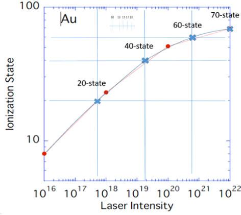
Figure 7: レーザー強度 W/\text{cm}^2 と金のイオン化状態。 ×印のレーザー強度がシミュレーションを行った値。
