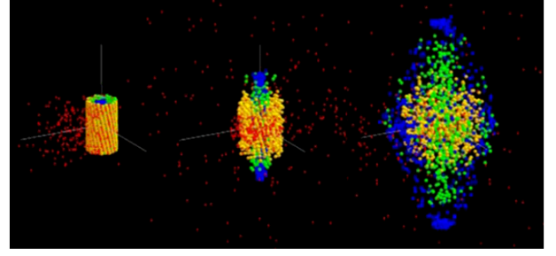
Figure 8: 電磁力によりナノチューブビームから噴き出す陽子・炭素・金イオンと電子のレーザー加速器。質量比は実際の値を用いており、電磁場は有限の幅を持つパルスで、レーザー強度は 7 \times 10^{17} \text{W}/\text{cm}^2 である。各時刻は t = 0, 4, 8 \text{ fs} である。
