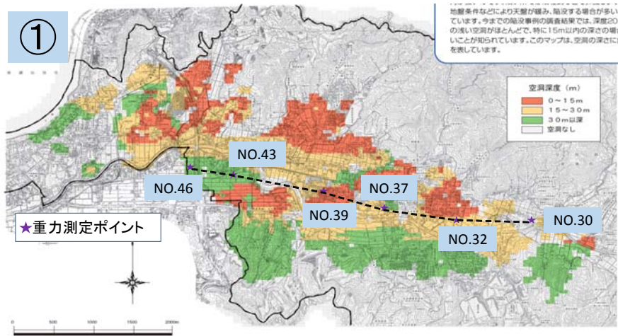
図-8 同一地質での重力測定地点
