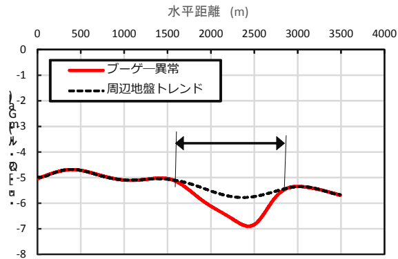
図-13 周辺地盤のトレンド
