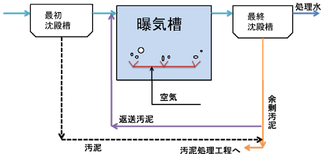
Fig.3 標準活性汚泥法の処理工程図
