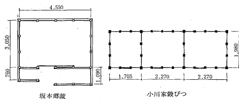
第2図 郷蔵平面図-II
