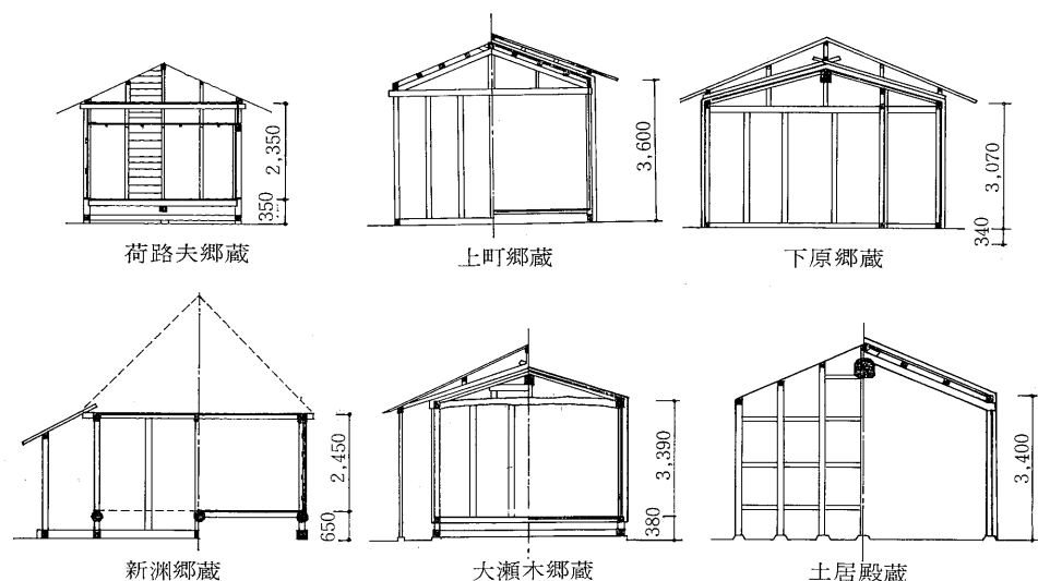
第3図 郷蔵断面図―Ⅰ
