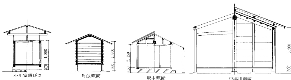
第4図 郷蔵断面図―Ⅱ
