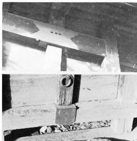
第10図 上町郷蔵帖木（出し入れ口の戸締り）
