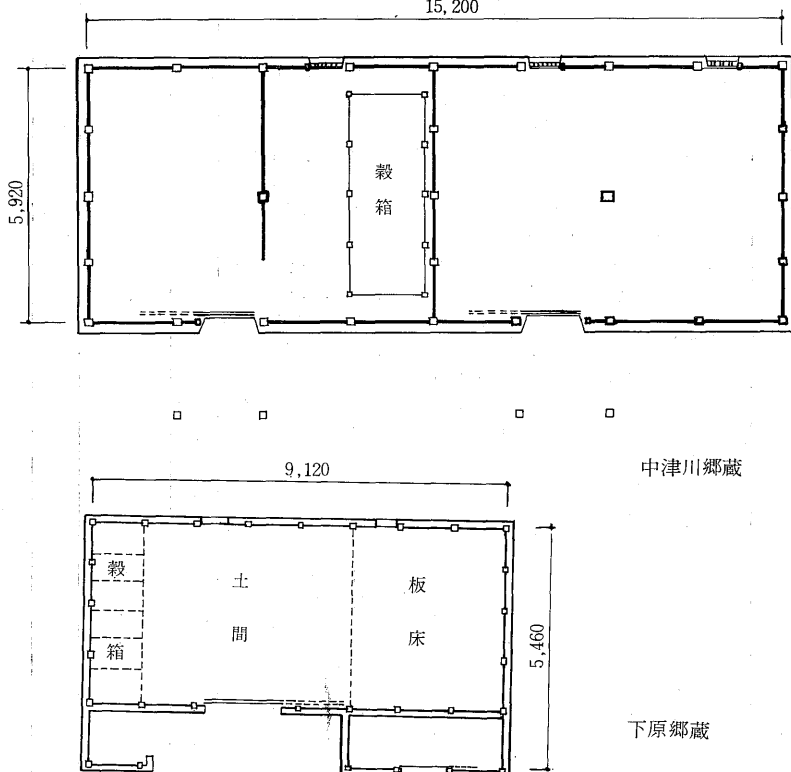
第1図 郷蔵平面図-I
